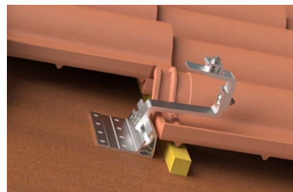
Dettaglio: gancio in alluminio GTA3.
